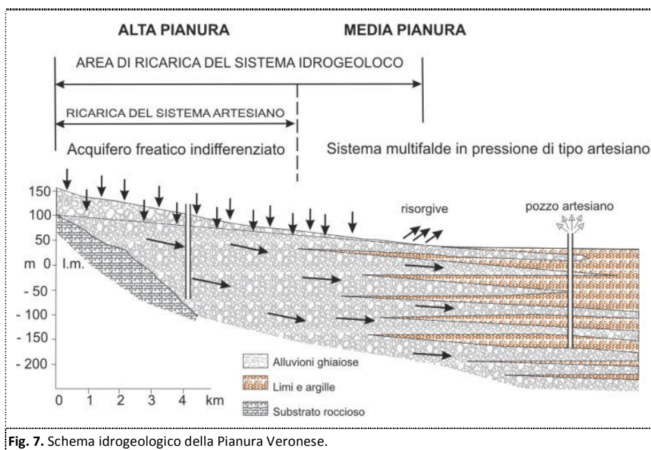
Fig. 7. Schema idrogeologico della Pianura Veronese.
